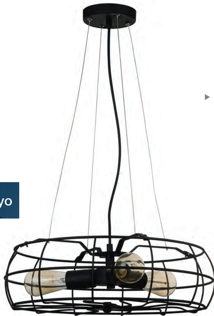
▲ MDM-2580/3 BK ø 45 x h. 14 / h. max 100 E27 3 x 60W
