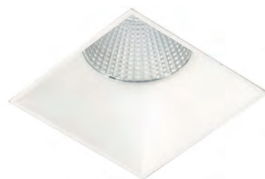
▲ SL74060/18W 3000K/4000K WH 12,5 x 12,5 x h. 12 LED 18W
