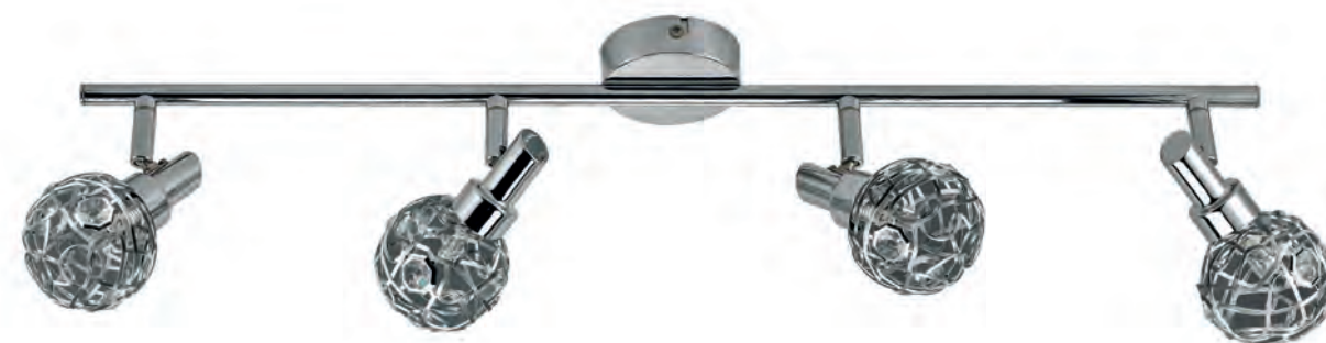
▲ HP-710AG-04-8008IUN 75 x 8 x h. 16,5 ☐ G9 4 x 28W
