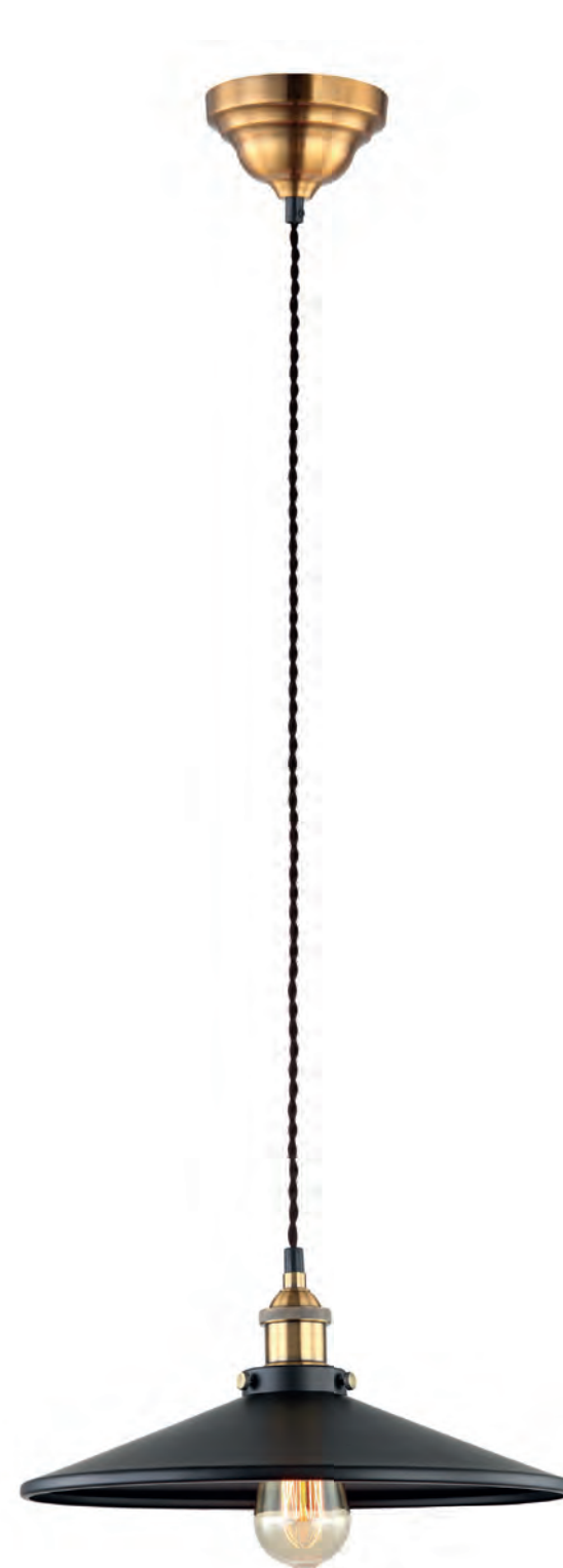
▲ MDM-3458/1L BK+GD ø 36 x h. max 94 E27 1 x 40W
