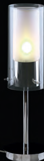
◀ MTM1851/1 ø 14 x h. 47 E14 1 x 40W
