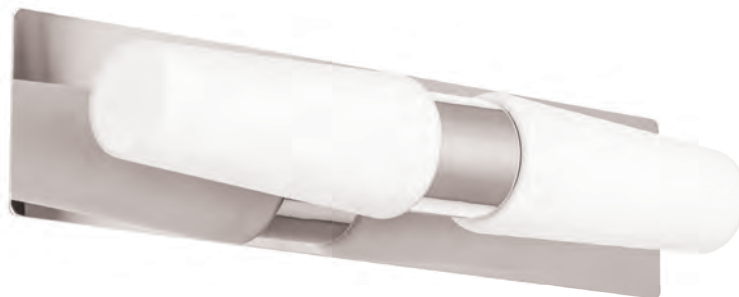
▲ MB12021106-2A 38 x 6,4 x h. 10,5 E14 2 x 40W IP44
