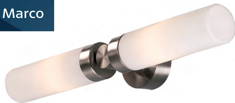
▲ MB4801-2A 40 x 7,4 x h. 9,5 G9 2 x 28W IP44
