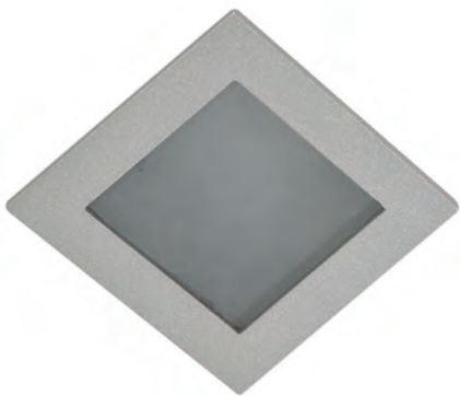
▲ DL-B01/SY 9 x 9 x h. 11,5 MR-16 1 x 35W
