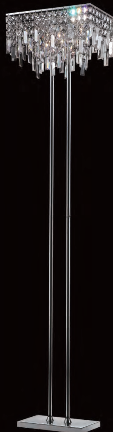
▼ ML92915-8B 38 x 24 x h. 162 ☐ G4 8 x 20W
