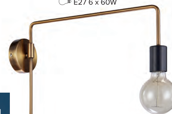
▼ MB-BR1721402-W1-G 59,5 x 48,5 x h. 10 E27 6 x 60W
