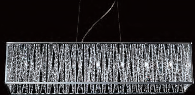
▲ P0282-07L-F4QL 86 x 25 x h. 18 / h. max 130 G9 7 x 42W
